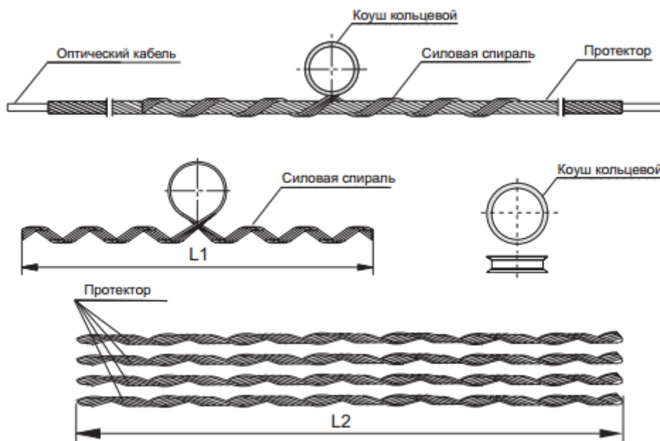
Рис.1. Зажим спиральный поддерживающий типа AXR-110
