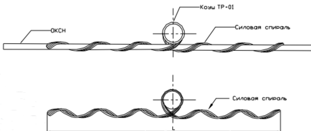
Рис.1. Зажим спиральный поддерживающий типа AX-50
